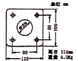
外形図
